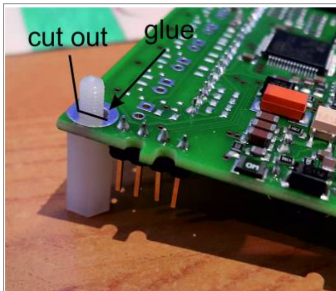
Option 1 - entretoises collé (photo SP9BSL)
