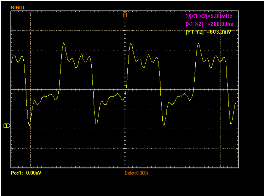
Pin 7 bei TX:
